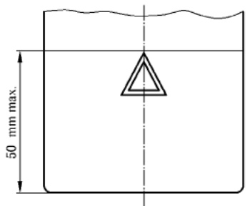
图3 带底包装触摸危险警示的位置
