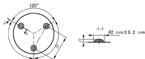
图 2 触摸危险警示的三点标志
